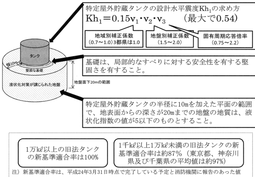
図-1 大規模石油タンク(旧法タンク)で講じられている地震対策の概要
