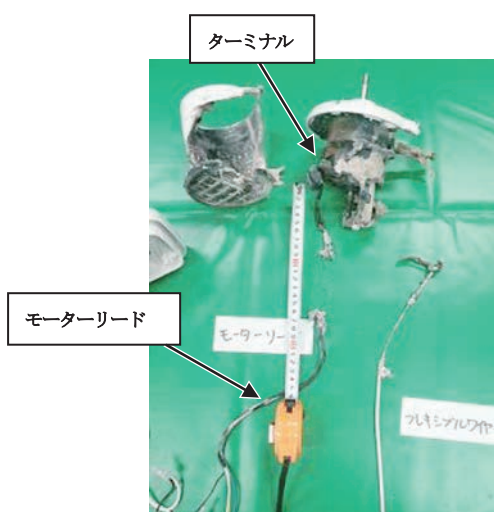
モーターリードの焼損状況
