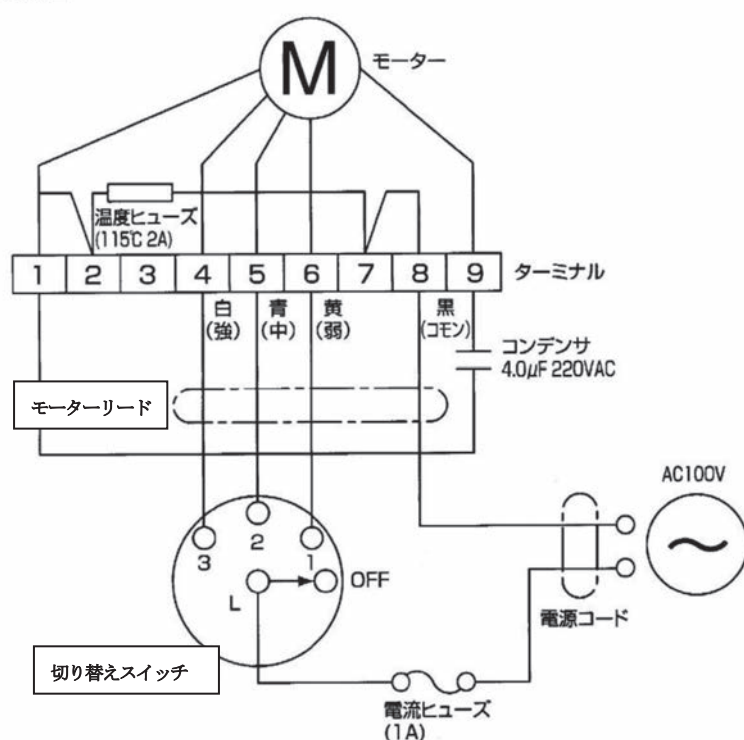
結線図
