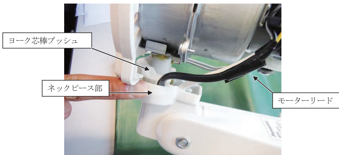
同型品のモーターリードの状況
