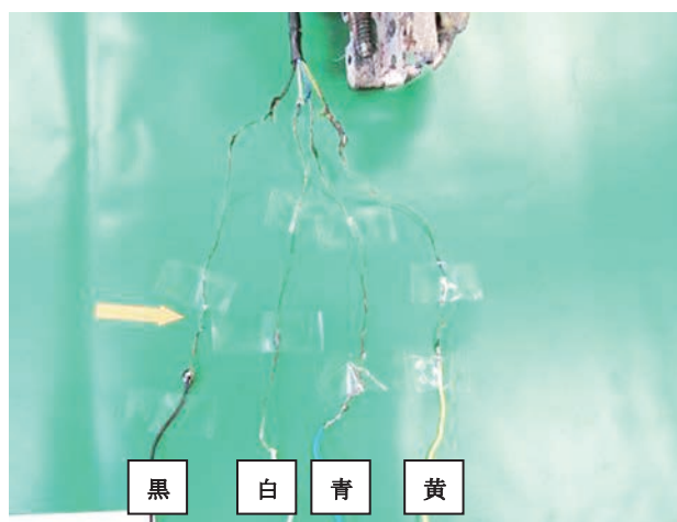
断線部分の状況
